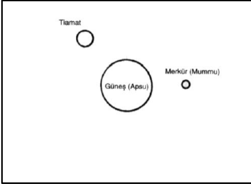
Şekil 102 – I. Başlangıçta: Güneş, Merkür, "Tiamat"
