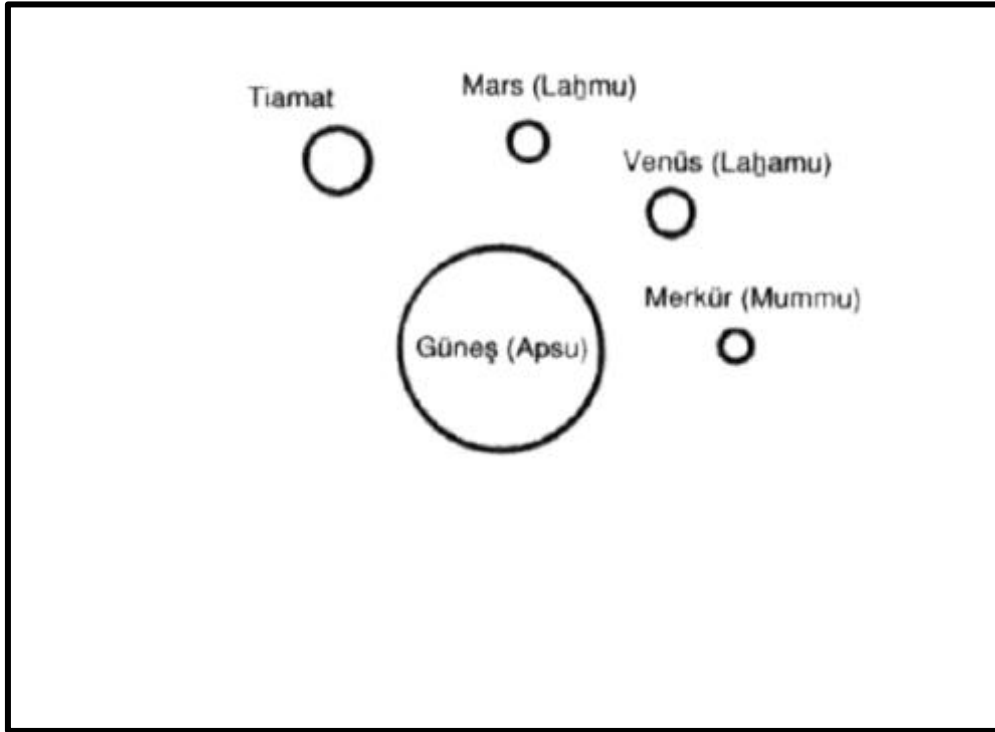
Şekil 103 – II. İçteki gezegenler, yani "Ortadaki tanrılar" doğar.
