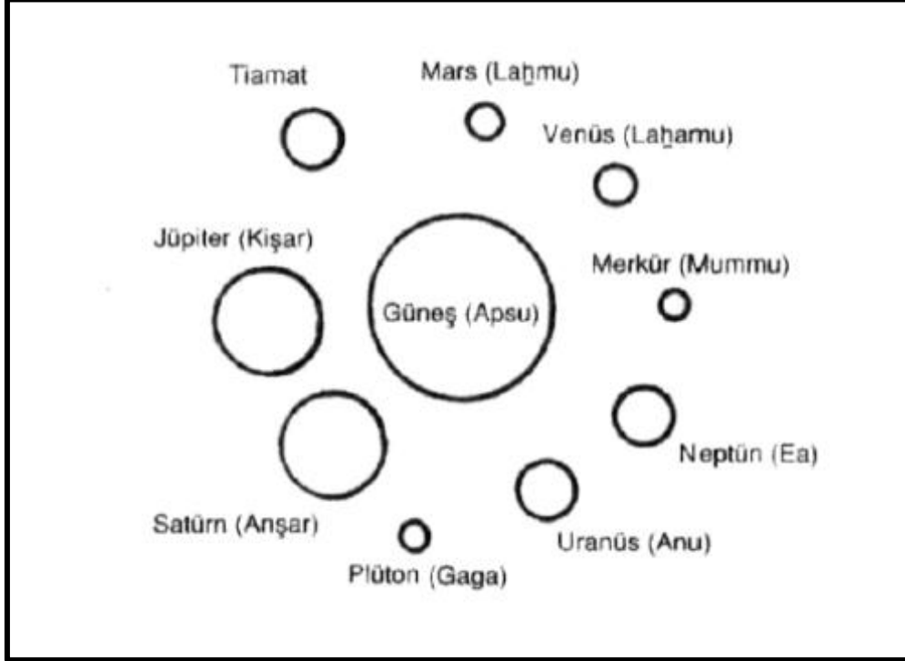
Şekil 105 – IV. Eşit, birbirinin suretinde olan son iki gezegen eklenir.
